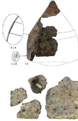
Resim 49: Semenovod’da Bulunan Miğfer Buluntusu. 1196
