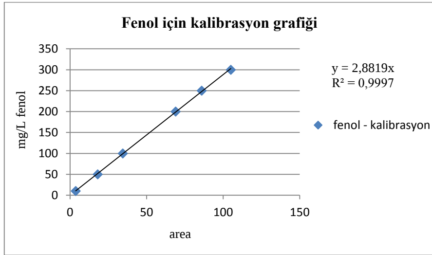
Şekil 16. HPLC’de yapılan fenol için konsantrasyon kalibrasyonu grafiği
