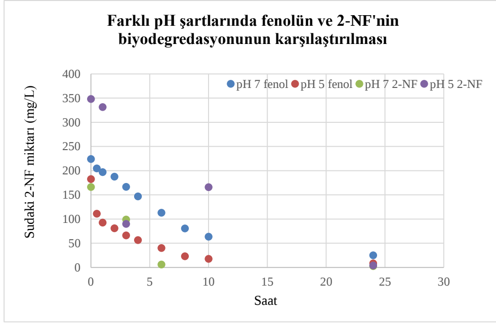
Şekil 33. 25°C’de ve pH 7 ve pH 5’te 1 U/mL dozda Lakkaz enziminin fenol ve 2-NF degradasyonu
