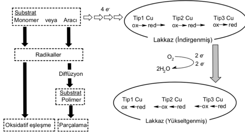
Şekil 3. Fungal lakkaz enzimlerinin reaksiyon mekanizmaları (Tuncer, 2010).
