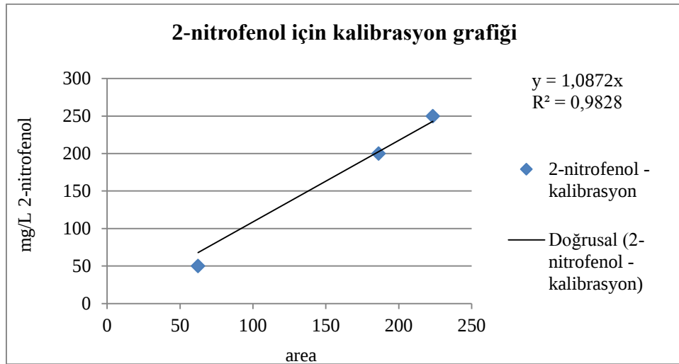
Şekil 18. HPLC’de yapılan 2-NF için konsantrasyon kalibrasyonu grafiği
