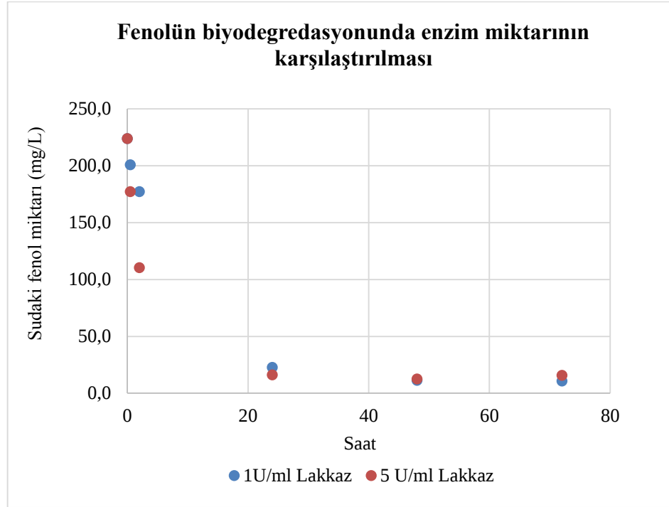
Şekil 23. 25 °C 1 U/mL ve 5 U/mL dozlarda Lakkaz enziminin fenol degradasyonu (Ph:7,2)
