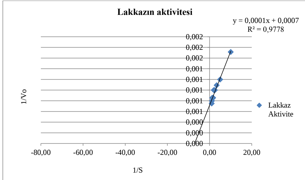
Şekil 15. ABST ile lakkaz enziminin aktivite tayininde elde edilen kalibrasyon eğrisi
