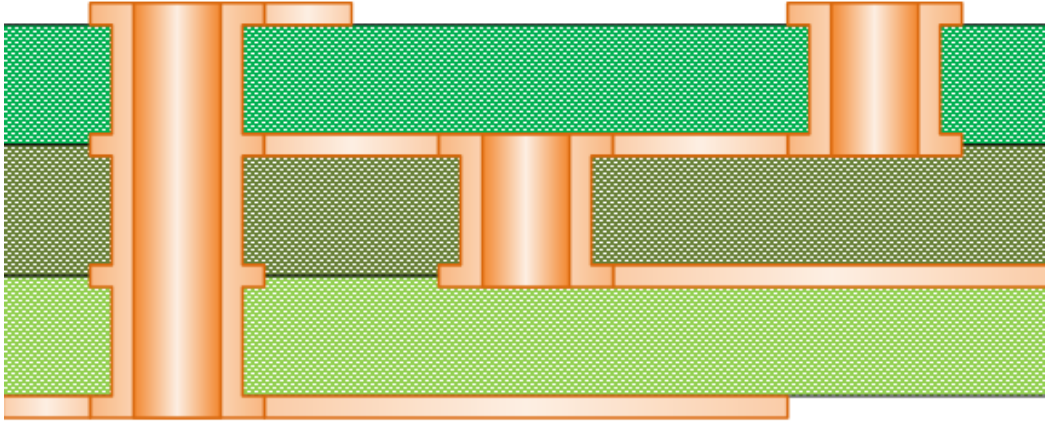
Şekil 22. Viaların PCB üzerindeki farklı yerleşimleri(Clinton, 2018).
