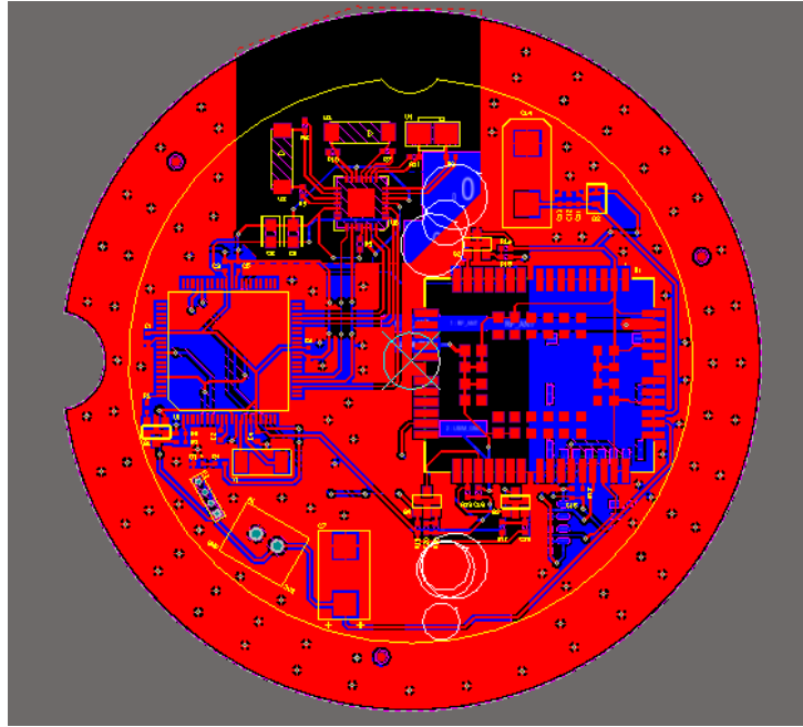
Şekil 24. PCB tasarımının son hali.
