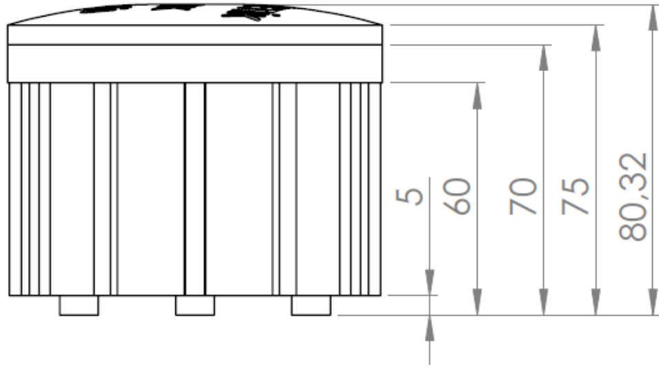
Şekil 30. Manyetik otopark sensörü kutusunun iki boyutlu tasarımı
