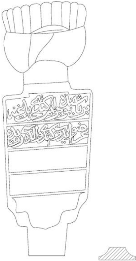
Çizim 120. Katalog B-23 Baş Şahidesi ve Gövde Yatay Kesiti
