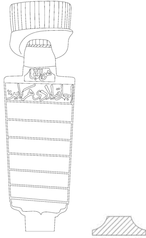
Çizim 36. Katalog A-36 Baş Şahidesi ve Gövde Yatay Kesiti
