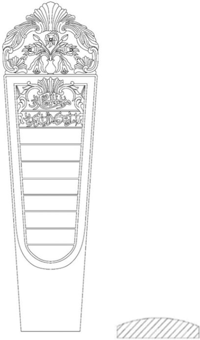
Çizim 69. Katalog A-73 Baş Şahidesi ve Gövde Yatay Kesiti
