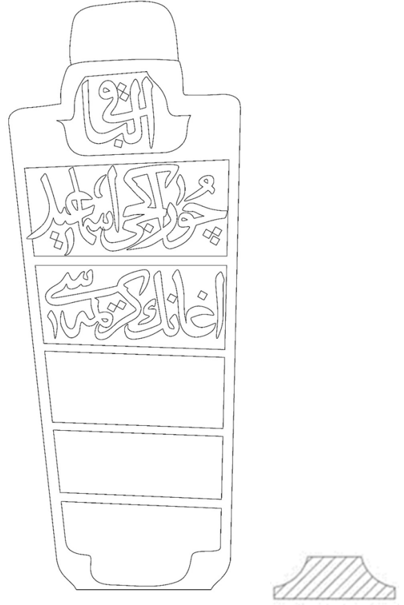
Çizim 22. Katalog A-22 Baş Şahidesi ve Gövde Yatay Kesiti
