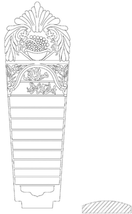
Çizim 81. Katalog A-85 Baş Şahidesi ve Gövde Yatay Kesiti
