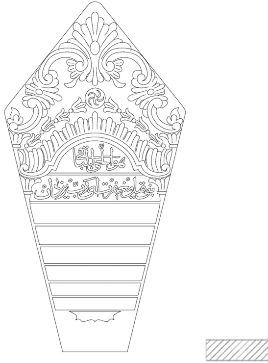
Çizim 128. Katalog B-31 Baş Şahidesi ve Gövde Yatay Kesiti
