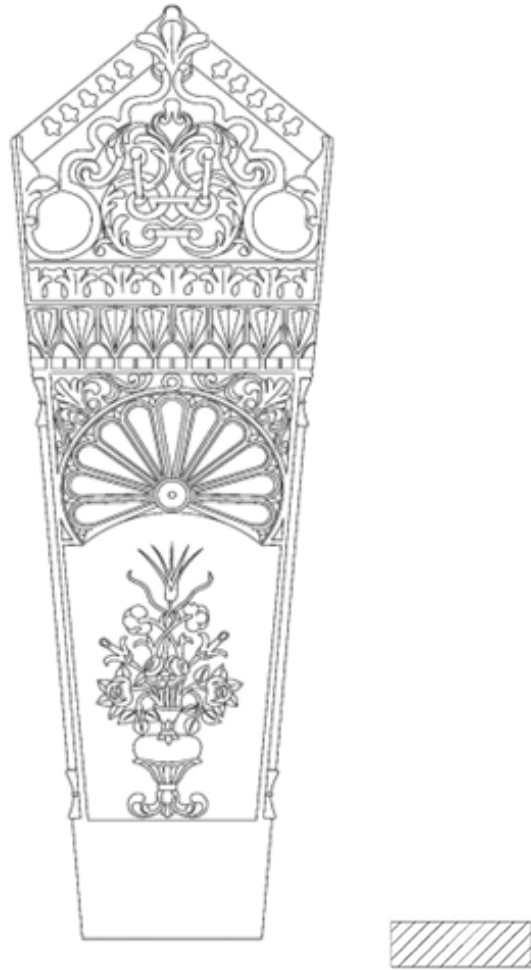
Çizim 105. Katalog B-8 Ayak Şahidesi ve Gövde Yatay Kesiti
