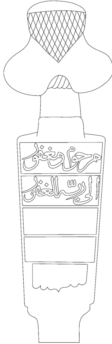
Çizim 137. Katalog B-40 Baş Şahidesi ve Gövde Yatay Kesiti
