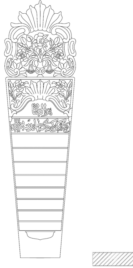
Çizim 39. Katalog A-39 Baş Şahidesi ve Gövde Yatay Kesiti
