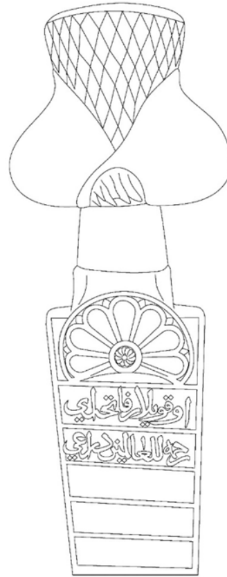
Çizim 125. Katalog B-28 Baş Şahidesi ve Gövde Yatay Kesiti
