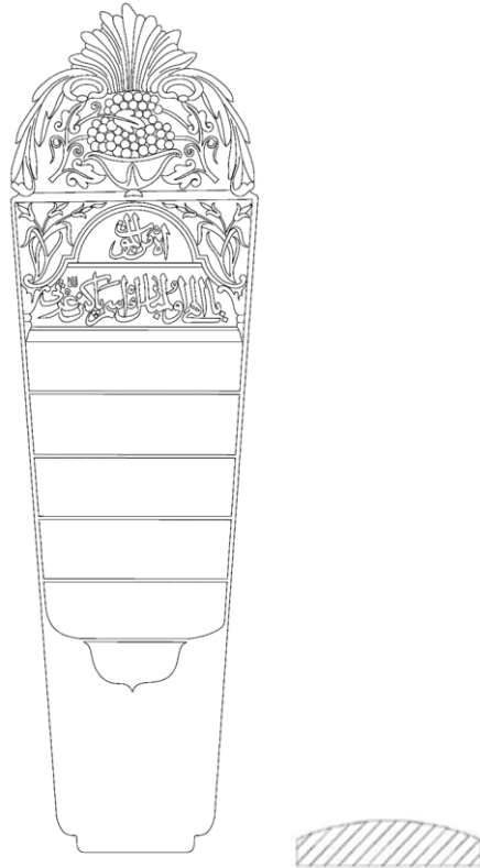
Çizim 63. Katalog A-66 Baş Şahidesi ve Gövde Yatay Kesiti
