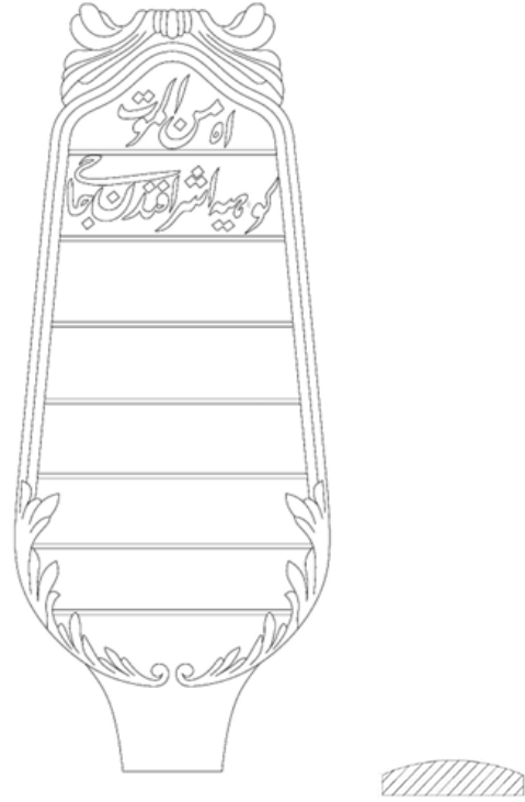
Çizim 83. Katalog A-87 Baş Şahidesi ve Gövde Yatay Kesiti
