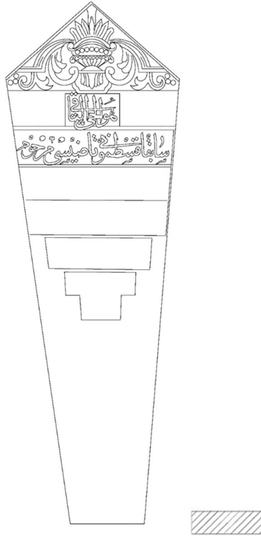
Çizim 102. Katalog B-5 Baş Şahidesi ve Gövde Yatay Kesiti
