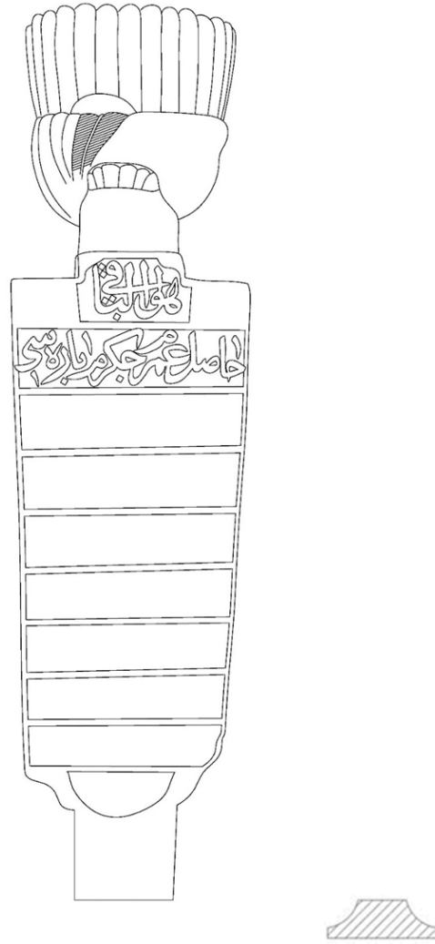
Çizim 119. Katalog B-22 Baş Şahidesi ve Gövde Yatay Kesiti
