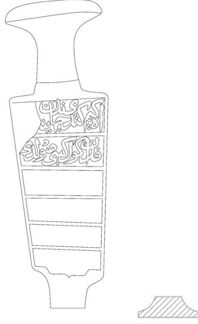
Çizim 114. Katalog B-17 Baş Şahidesi ve Gövde Yatay Kesiti
