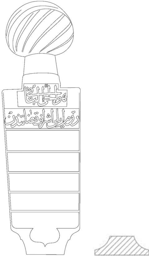
Çizim 9. Katalog A-9 Baş Şahidesi ve Gövde Yatay Kesiti
