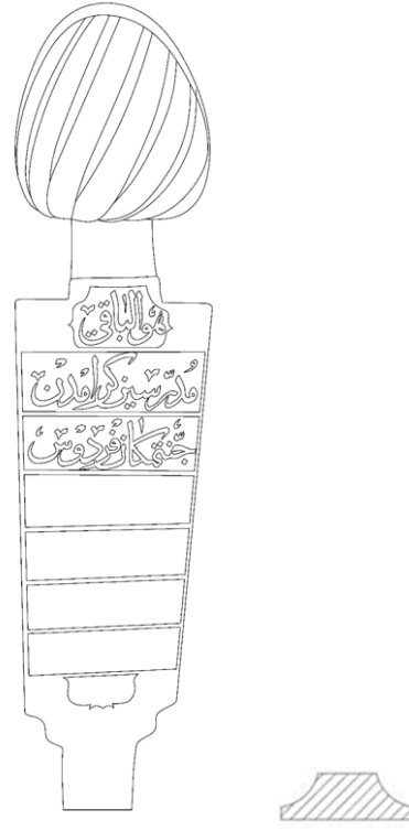
Çizim 78. Katalog A-82 Baş Şahidesi ve Gövde Yatay Kesiti
