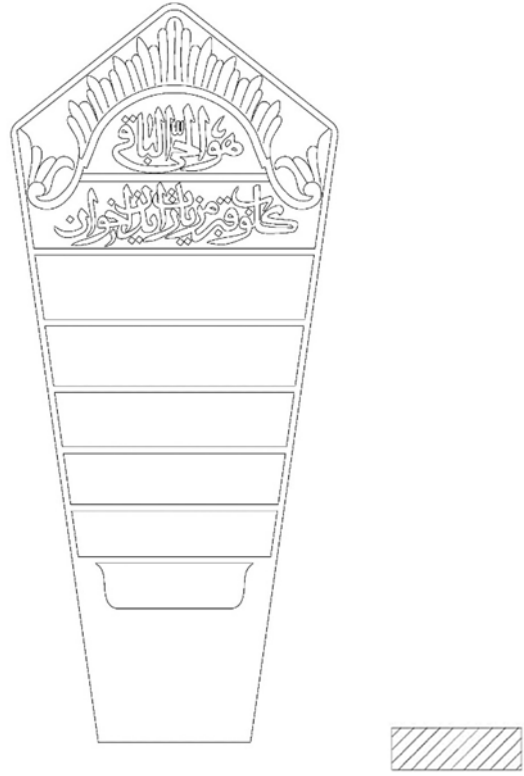
Çizim 122. Katalog B-25 Baş Şahidesi ve Gövde Yatay Kesiti
