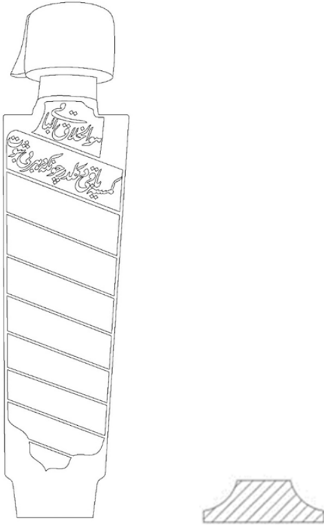
Çizim 16. Katalog A-16 Baş Şahidesi ve Gövde Yatay Kesiti
