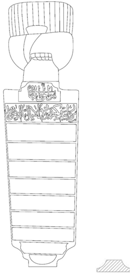
Çizim 110. Katalog B-13 Baş Şahidesi ve Gövde Yatay Kesiti
