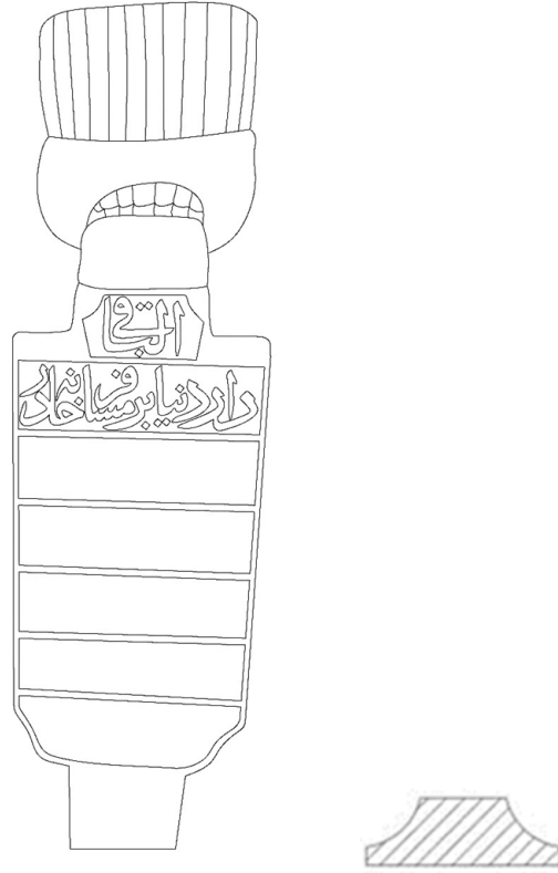
Çizim 34. Katalog A-34 Baş Şahidesi ve Gövde Yatay Kesiti
