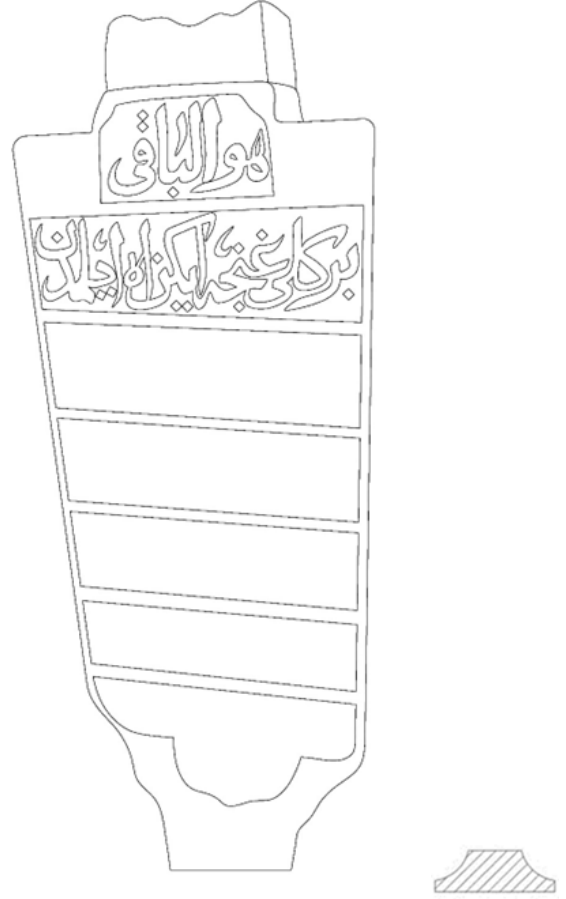
Çizim 87. Katalog A-91 Baş Şahidesi ve Gövde Yatay Kesiti
