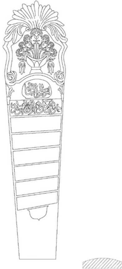
Çizim 98. Katalog B-1 Baş Şahidesi ve Gövde Yatay Kesiti
