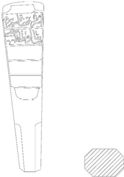
Çizim 19. Katalog A-19 Baş Şahidesi ve Gövde Yatay Kesiti
