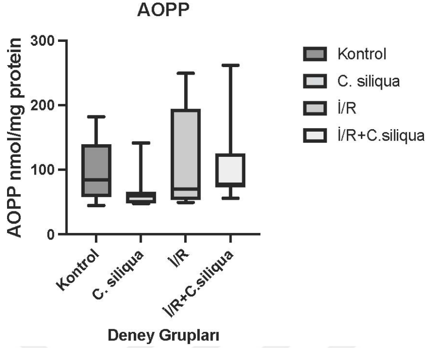
Şekil 4.84: Gruplar arası AOPP seviyelerinin karşılaştırılması. Anlamli farklılık saptanmamıştır. Değerler medyan ve IQR olarak verilmiştir.
