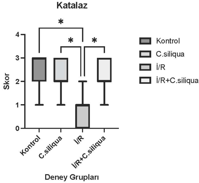
Şekil 4.56: Katalaz skorlaması. Anlamlı farklılık düzeyi (*) gösterilmektedir. Değerler medyan ve IQR olarak ifade edilmiştir. (*: p<0.05 )
