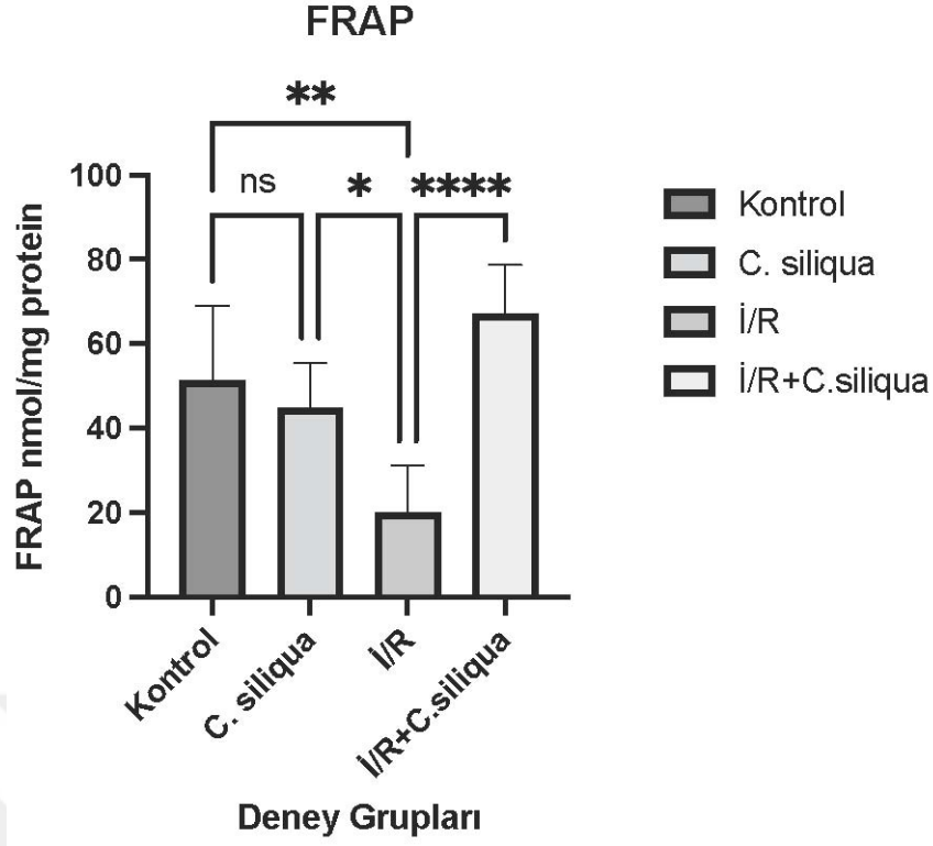
Şekil 4.85: Gruplar arası FRAP seviyelerinin karşılaştırılması. Anlamlı farklılık düzeyi (*), (**) ve (***) olarak gösterilmektedir. Değerler ortalama ve SD olarak verilmiştir. (*: p<0.05 ; **: p<0.01 ; ***: p<0.001 )
