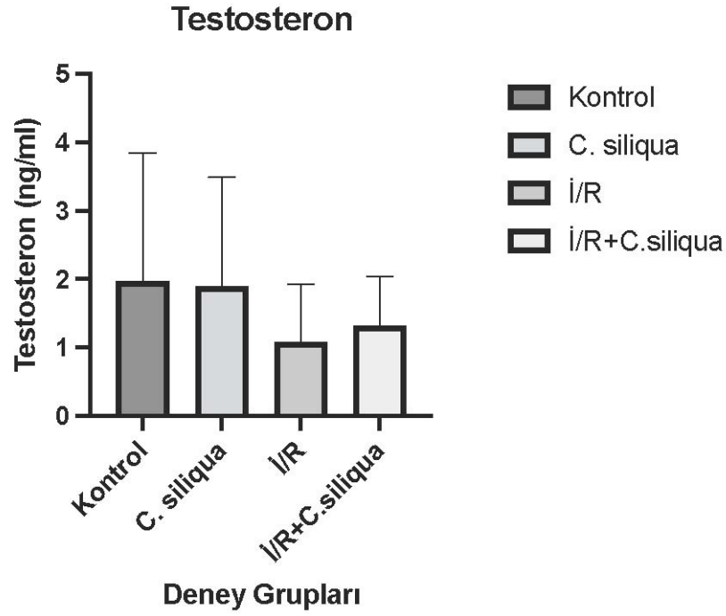
Şekil 4.86: Gruplar arası serum testosteron düzeylerinin karşılaştırılması. Anlamli farklılık saptanmamıştır. Değerler ortalama ve SD olarak verilmiştir.
