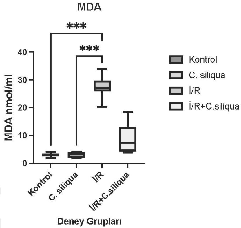
Şekil 4.82: Gruplar arası MDA seviyelerinin karşılaştırılması. Anlamlı farklılık düzeyi (***) olarak gösterilmektedir. Değerler medyan ve IQR olarak verilmiştir. (***: p<0.001 )
