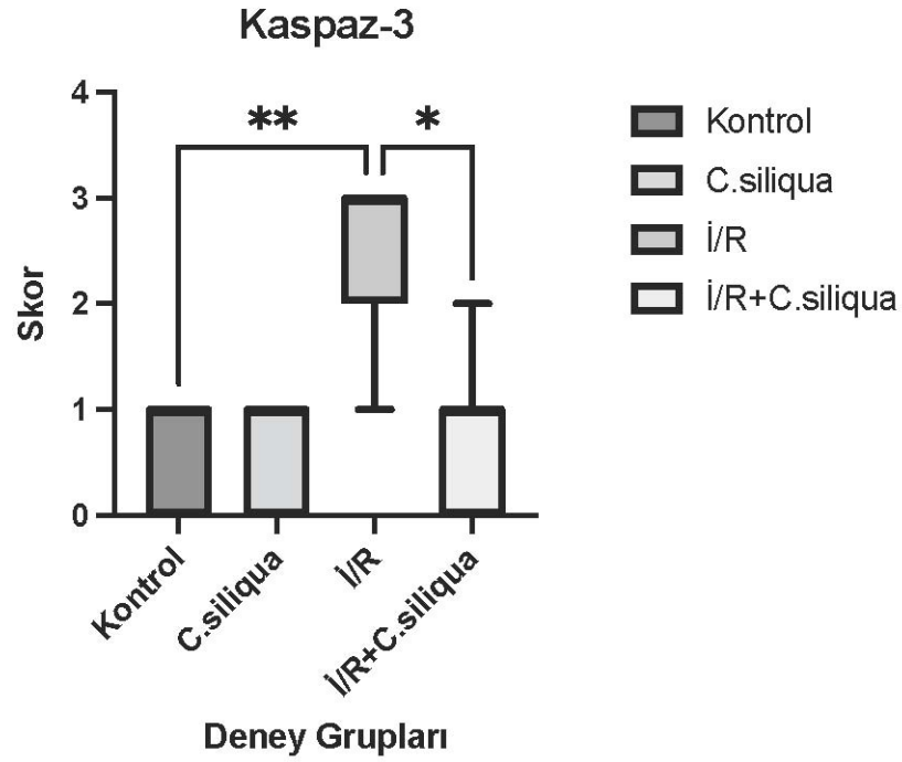
Şekil 4.28: Kaspaz-3 skorlaması. Anlamlı farklılık düzeyi (*) ve (**) gösterilmektedir. Değerler medyan ve IQR olarak ifade edilmiştir. (*: p<0.05 ; **: p<0.01 )
