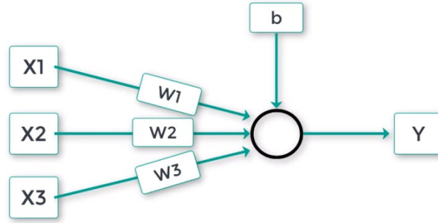
Şekil 3.3 Derin Sinir Ağına Ait Nöron Yapısı
