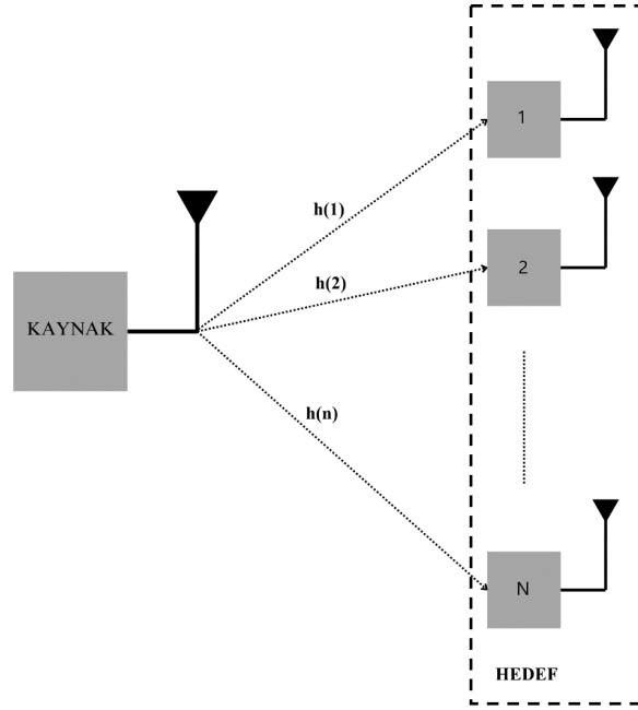
Şekil 2.1 Bir Kaynak, N Adet Hedeften Oluşan Kablosuz Haberleşme Modeli (SIMO)
