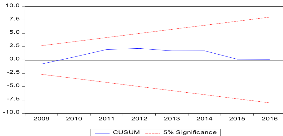
Fig. 4. CUSUM.
