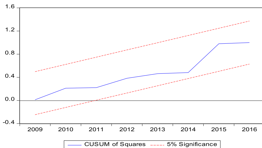
Fig. 3. CUSUMSQR.
