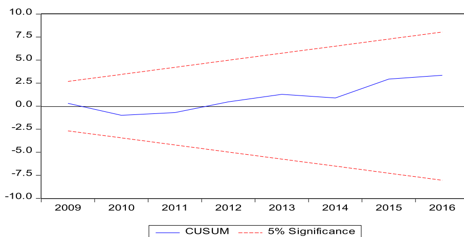
Fig. 2. CUSUM.
