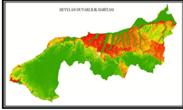
Harita 5: Yalova ili heyelan duyarlık haritası
